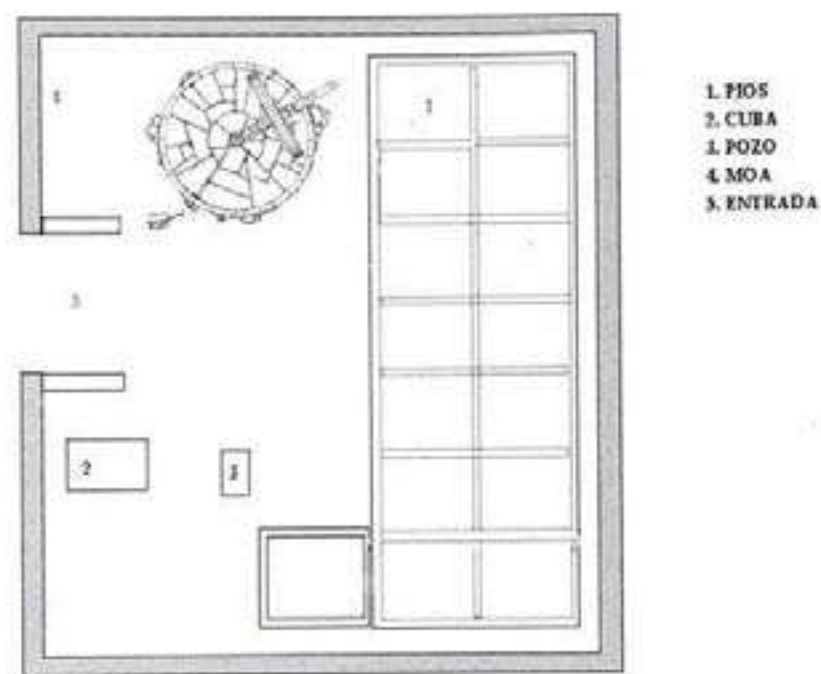
Esquema da Atahona das Testeiras
